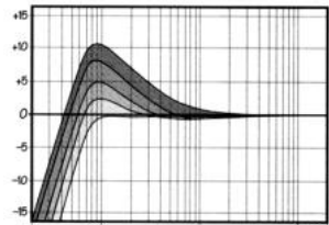
Низкочастотная эквалайзация с обрезным фильтром
