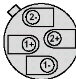
Рисунок 9. Разъем динамика
