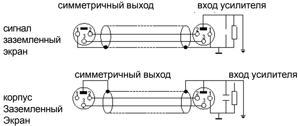
Рисунок 6. Симметричная линия
