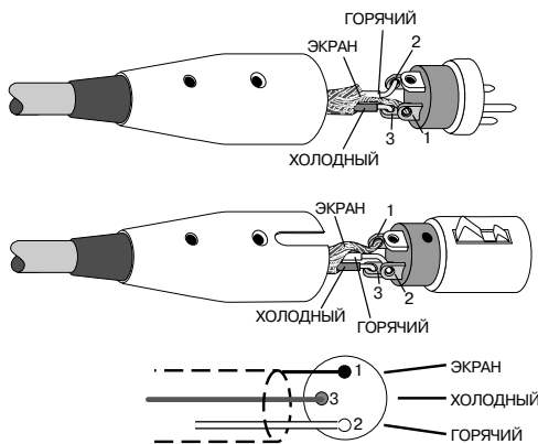
Разъем XLR
